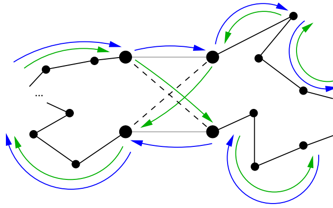
Figura 10.1: Una modificación 2-opt para el problema del viajante: la ruta original R está marcada por las flechas azules y la ruta más económica R' por las flechas verdes; las aristas eliminadas están en gris y las añadidas en línea negro discontinua. Los cuatro vértices que son puntos finales de las aristas involucradas están dibujados en mayor tamaño que los otros vértices.
