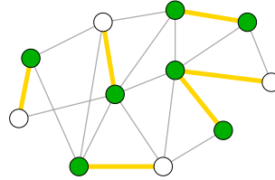
Figura 4.3: Ejemplos de cubiertas: los vértices verdes cubren todas las aristas y las aristas amarillas cubren todos los vértices.
