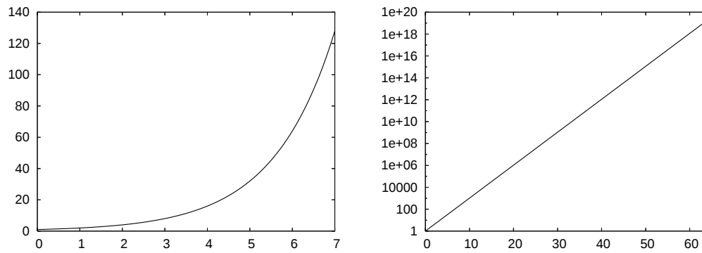
Figura 1.3: Gráficas de las potencias de dos: a la izquierda, con ejes lineales hasta x = 7 , y a la derecha, con ejes de escala logarítmica hasta x = 64 .
