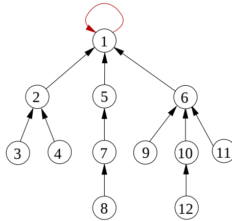
Figura 6.17: Un ejemplo de los punteros padre de un árbol con n claves posibles para poder guardar su estructura en un arreglo de tamaño n .
